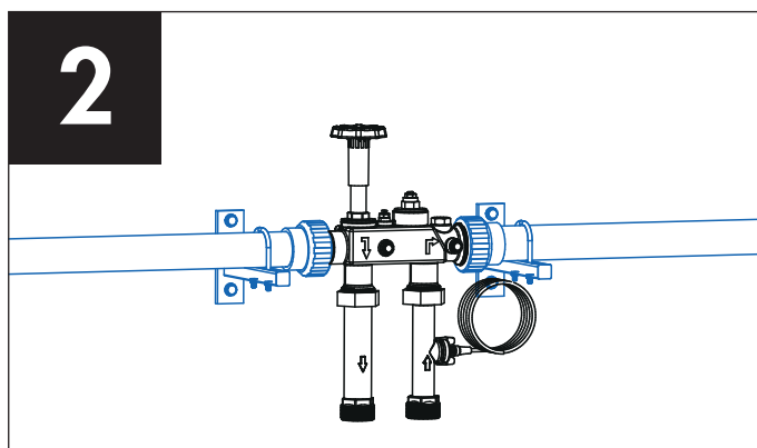
2 Mise en place du module de raccordement S.C.
