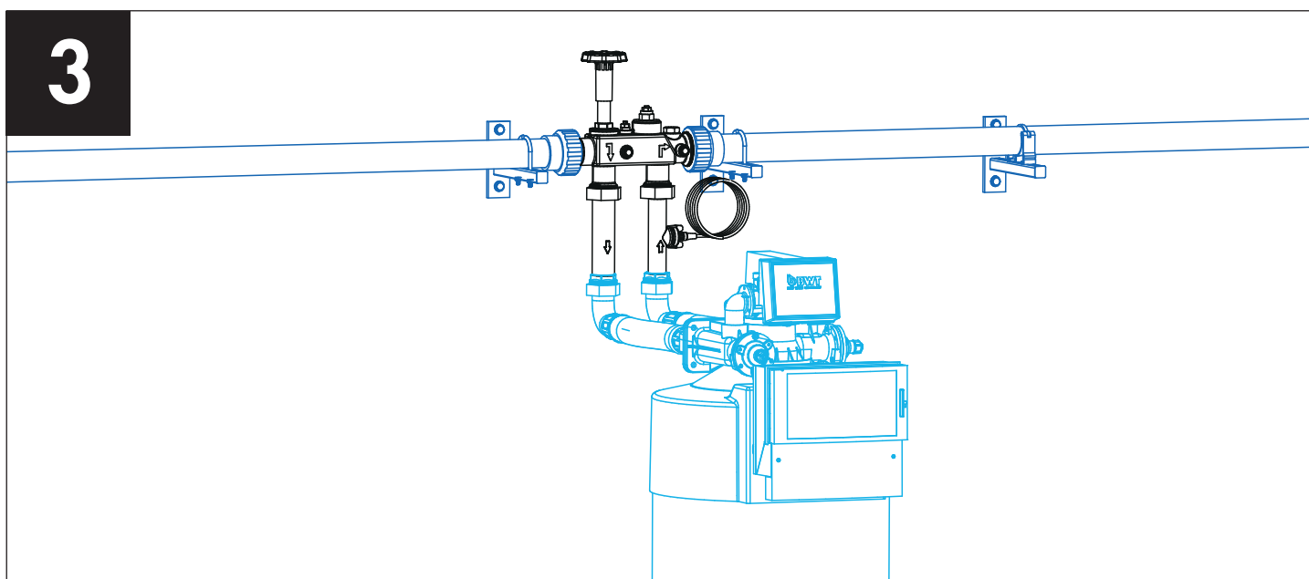
3 Raccordement de l'adoucisseur simplyconnect et mise en service.
